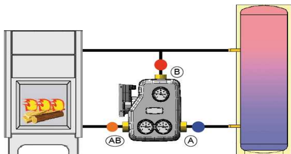
Монтаж вдясно от котела.
