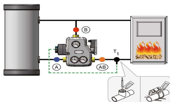
Монтаж вляво от котела.
