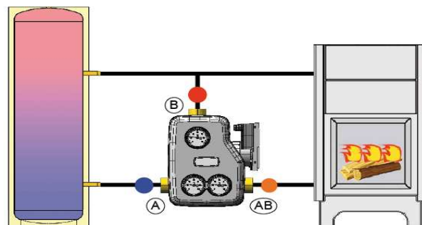
Монтаж вляво от котела.
