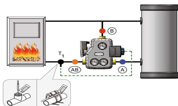
Монтаж вдясно от котела.
